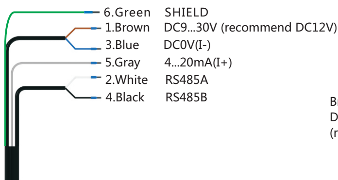
Electrode outlet
